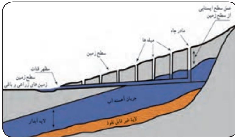
شکل ۱۲- نیمرخ قنات
