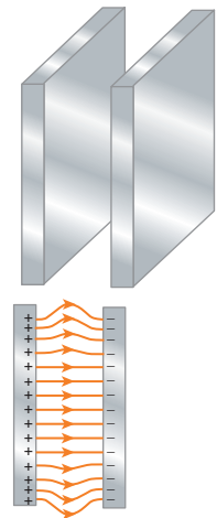
شکل ۲۰-۱ طرحی از خطوط میدان یکنواخت بین دو صفحه رسانای موازی با بارهای هم‌اندازه و ناهمنام
