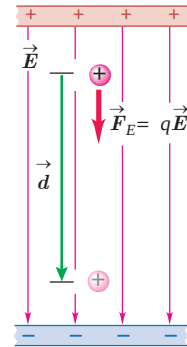
شکل ۷-۲ ذره باردار q در میدان الکتریکی یکنواخت رها می شود و به تدریج بر انرژی جنبشی آن افزوده می شود (از نیروی گرانشی چشم پوشی شده است).
