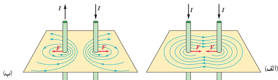
شکل ۳-۱۶ نیروی بین دو سیم موازی حامل جریان و رسم خطوط میدان مغناطیسی برایتد آنها. الف) برای جریان‌های همسو، راباشی است و ب) برای جریان‌های ناهمسو، رانشی است.
