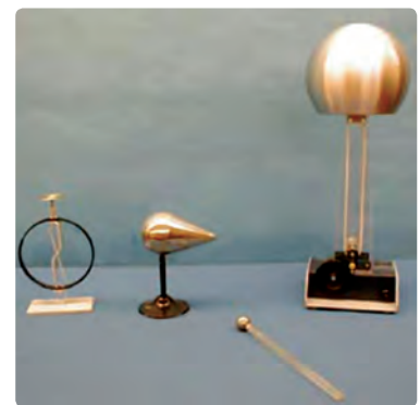
شکل ۱-۲۸ اسباب آزمایش چگونگی توزیع بار روی سطح خارجی یک جسم رسانای باردار
