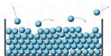
شکل ۴-۲۳ در حین تبخیر سطحی، مولکول‌های پراورزی‌تر از سطح مایع می‌گریزند.
