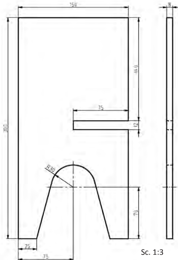
شکل ۶-۳۰- نقشه پروژه رحل قرآن
